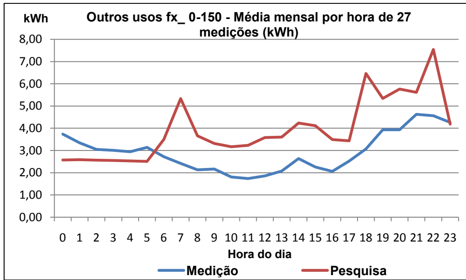
Figura 5.15 - Curvas de cargas médias mensais declaradas e medidas (hxh) para Outros usos Fx_0-150 kWh - 27 casos
