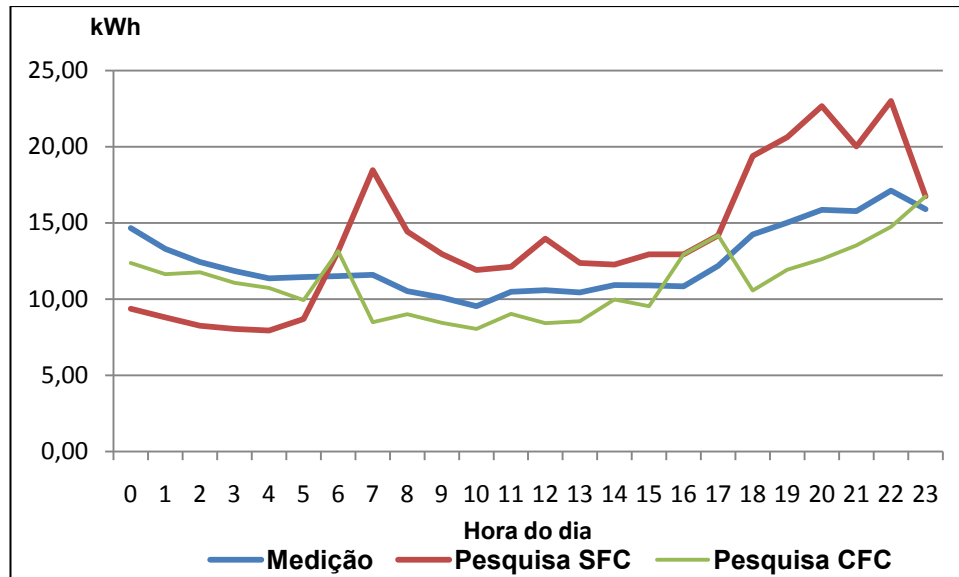
Figura 5.50 - Curvas de cargas médias mensais declaradas, medidas, declaradas CFC (SOLVER) (hxh) para Todos os aparelhos – 120 clientes
