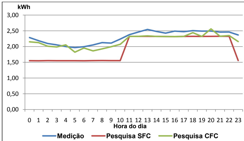
Figura 5.24 - Curvas de cargas médias mensais declaradas, medidas, declaradas CFC (2 parâmetros) (h xh ) para geladeiras – 124 casos
