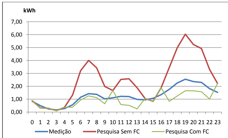
Figura 5.40 - Curvas de cargas médias mensais declaradas MM3, medidas MM3, declaradas CFC MM3 (SOLVER) (h/h) para Chuveiro – 58 casos
