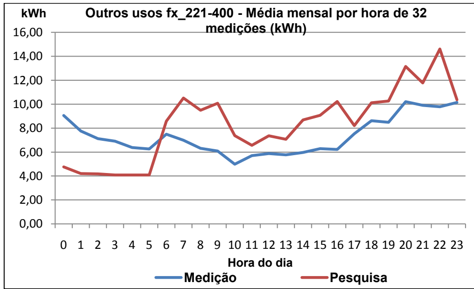
Figura 5.17 - Curvas de cargas médias mensais declaradas e medidas (hxx) para Outros usos Fx_221-400 kWh - 32 casos
