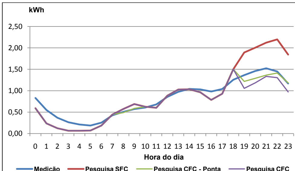
Figura 5.34 - Curvas de cargas médias mensais declaradas, medidas, declaradas CFC (SOLVER), declaradas CFC-ponta (SOLVER) (hxh) para Televisores – 160 casos.
