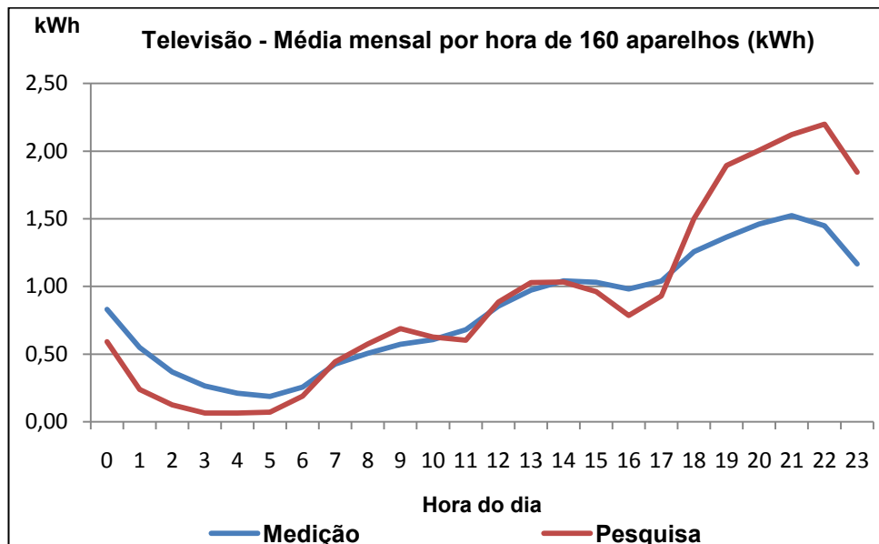
Figura 5.11 - Curvas de cargas médias mensais declaradas e medidas (hxh) para Televisor - 160 casos
