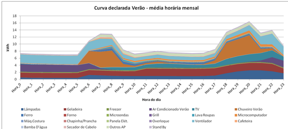
Figura 5.52 - Curvas de cargas médias mensais declaradas (hxh) para um cliente Ampla - verão
