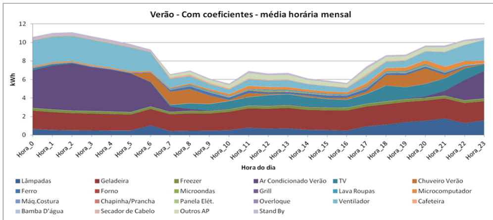
Figura 5.53 - Curvas de cargas médias mensais declaradas CFC (SOLVER) (hxh) para um cliente Ampla – verão.
