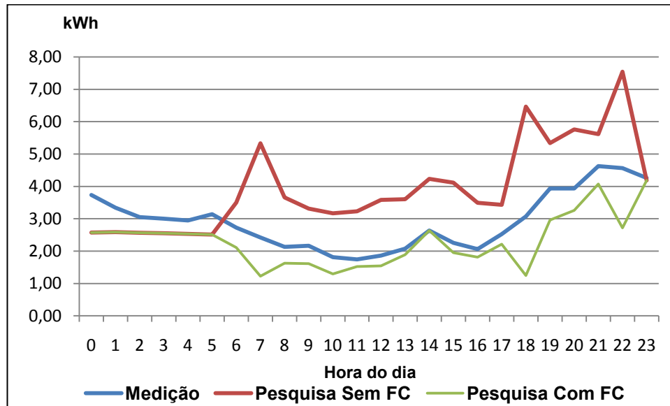
Figura 5.42 - Curvas de cargas médias mensais declaradas, medidas, declaradas CFC (SOLVER) (hxh) para Outros usos fx 0-150kWh – 27 casos.
