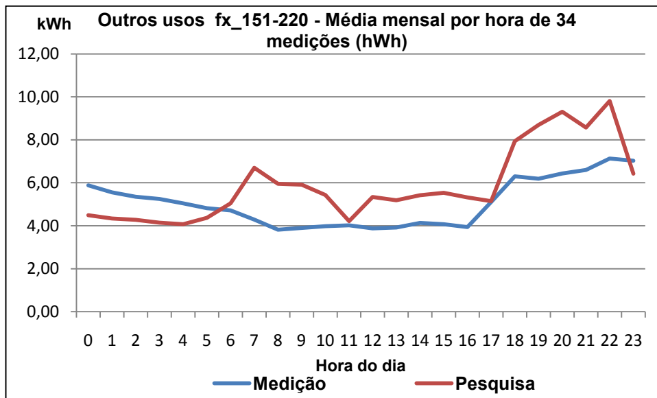
Figura 5.16 - Curvas de cargas médias mensais declaradas e medidas (hxh) para Outros usos Fx_151-220 kWh - 34 casos
