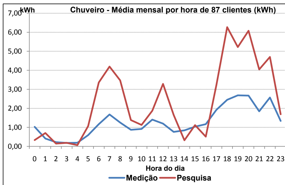
Figura 5.14 - Curvas de cargas médias mensais declaradas e medidas (hxh) para Chuveiro - 87 casos
