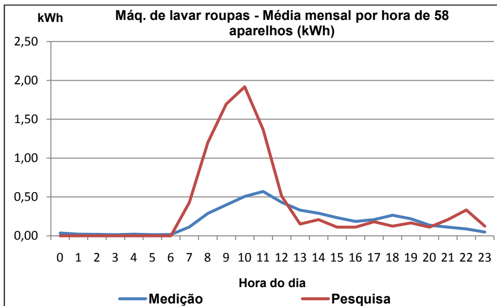
Figura 5.12 - Curvas de cargas médias mensais declaradas e medidas (hxh) para Máquina de lavar - 58 casos
