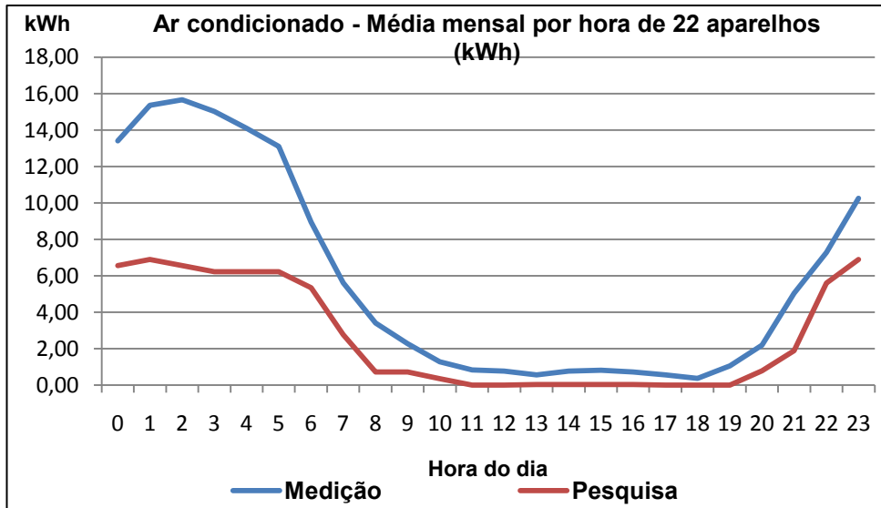
Figura 5.13 - Curvas de cargas médias mensais declaradas e medidas (hxh) para Ar condicionado - 22 casos
