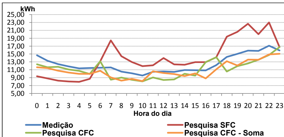
Figura 5.51 - Curvas de cargas médias mensais declaradas, medidas, declaradas CFC (SOLVER), declaradas CFC-Soma (SOLVER) (hxx) – 120 clientes
