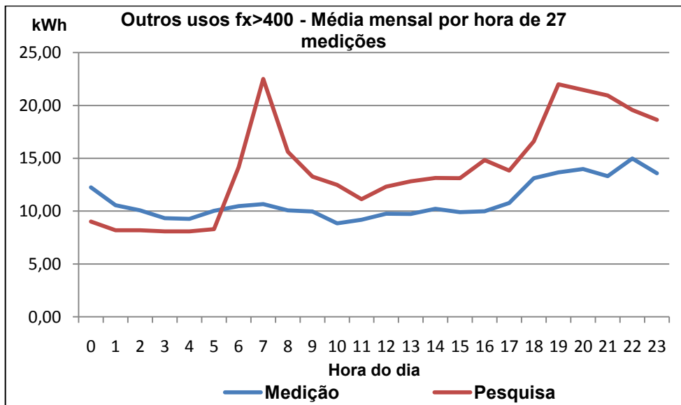
Figura 5.18 - Curvas de cargas médias mensais declaradas e medidas (hxx) para Outros usos Fx>400 kWh - 27 casos
