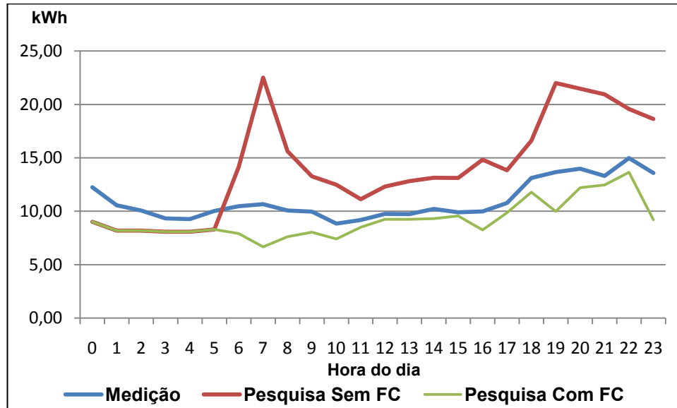
Figura 5.48 - Curvas de cargas médias mensais declaradas, medidas, declaradas CFC (SOLVER) (hxh) para Outros usos fx >400kWh – 27 casos
