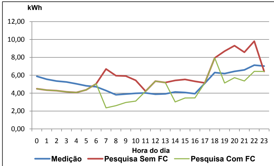
Figura 5.44 - Curvas de cargas médias mensais declaradas, medidas, declaradas CFC (SOLVER) (hxh) para Outros usos fx 151-220 kWh – 34 casos
